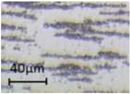
磁場付与によるMTMFのクラスター構造
