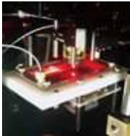
本研究で開発中のマイクロ空間ラマン分光システム
