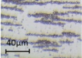
磁場付によるMTMFのクラスター構造
