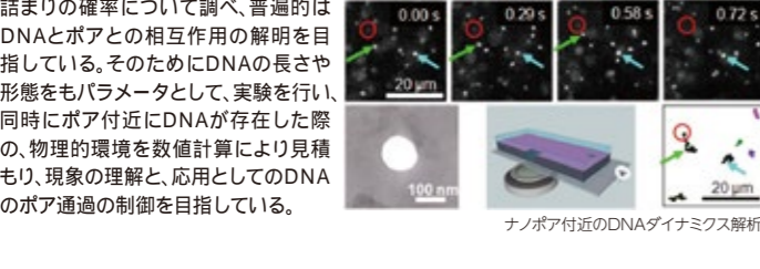
ナノポア付近のDNAダイナミクス解析
